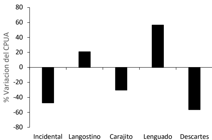
Fig. 14. Variación de la CPUA promedio (%) obtenido con la red modificada con ventana chica (RM-I) en relación a la red convencional (RC) en los lances de comparación en la pesca de arrastre de langostino.
