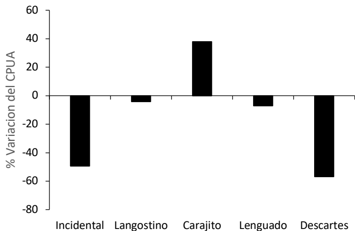
Fig. 15. Variación de la CPUA promedio (%) obtenido con la red modificada con ventana grande (RM-II) y la red convencional (RC) registrada en los lances de comparación en la pesca de arrastre de langostino.
