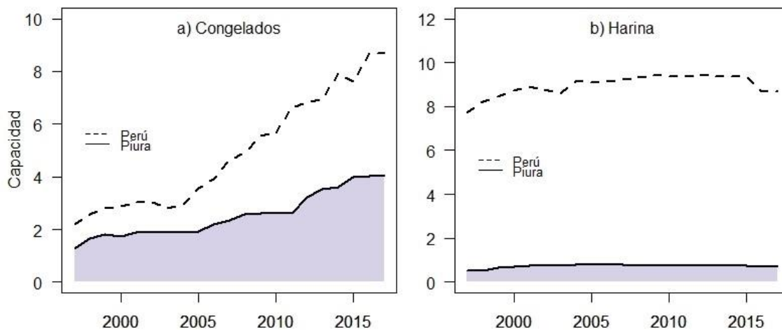
MS Figura 2: Desarrollo de la capacidad de producción en Piura y en todo el Perú entre 1997 y 2017 de a) congelados (miles de toneladas de recepción de materia prima al día) y b) harina de pescado (miles de toneladas de recepción por hora).
